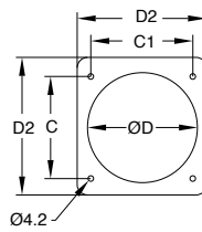
Ölçüler (mm)
